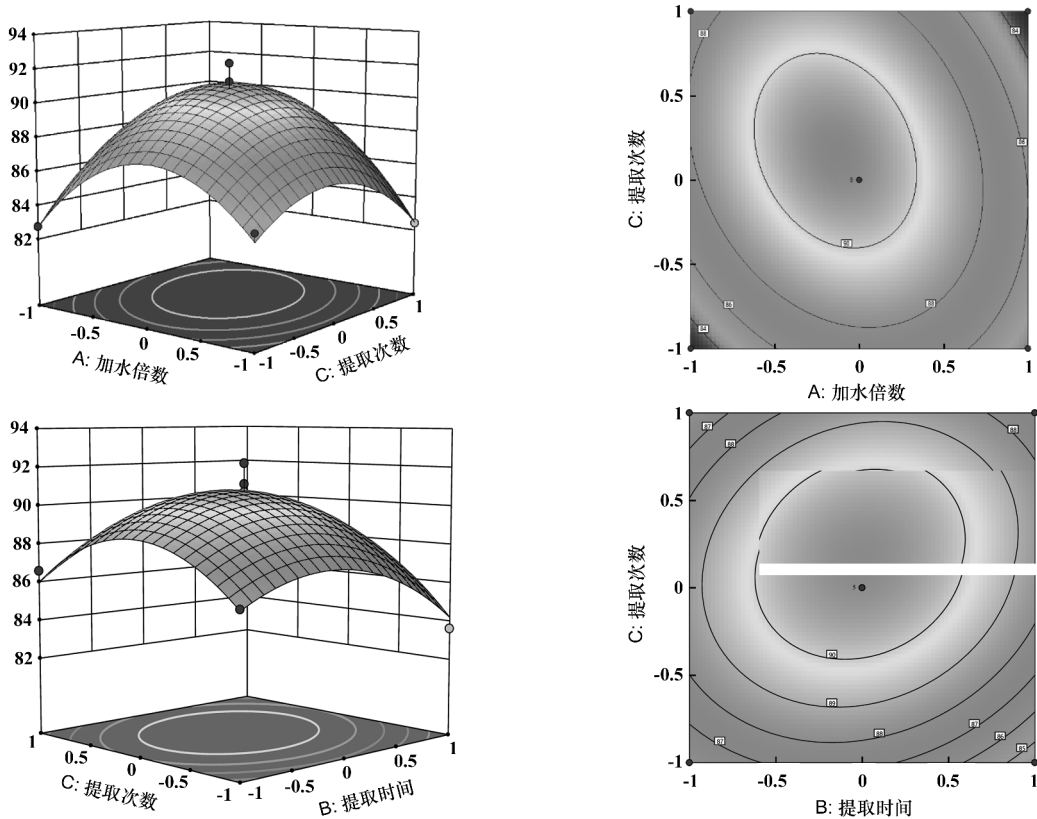
图 2 各因素交互作用 3D 曲面图和等高线图
