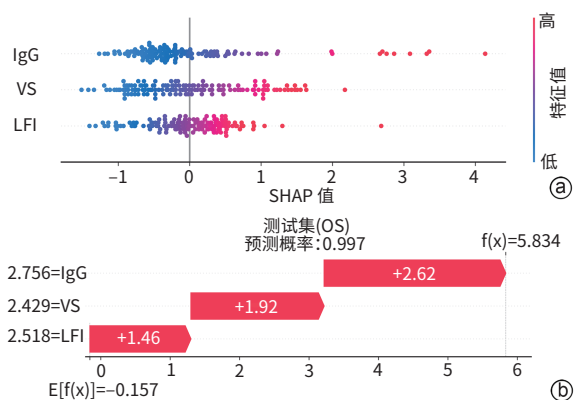
注:a,SHAP摘要图;b,测试集中1例患者的预测过程。IgG,免疫球蛋白G;VS,剪切波速度;LFI,肝纤维化指数;OS,重叠综合征;LR,逻辑回归;SHAP,沙普利加性解释。
