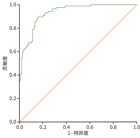
图4 建模组的受试者操作特征曲线
