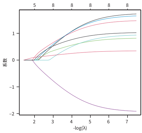
图1 LASSO回归系数关系
