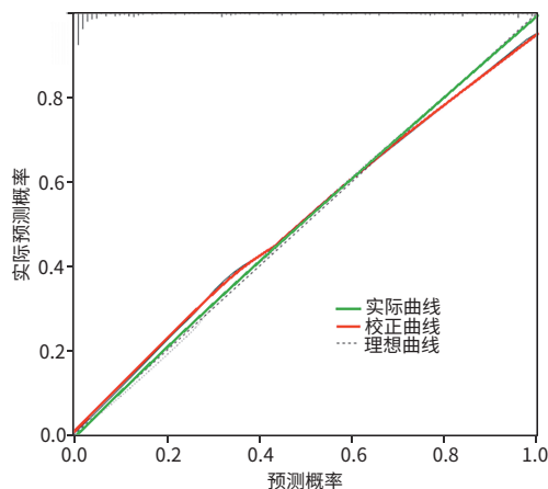
图5 建模组的校准曲线
