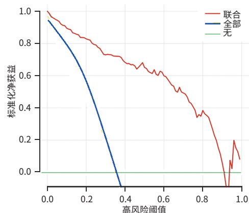
图8 列线图模型的决策曲线分析
