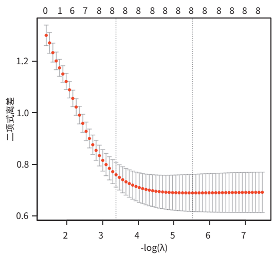
图2 10折交叉验证LASSO回归降维图
