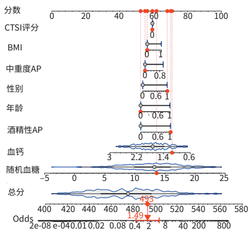
图3 PPDM-A的列线图模型
