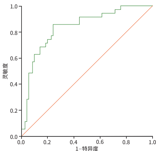
图6 验证组的受试者操作特征曲线
