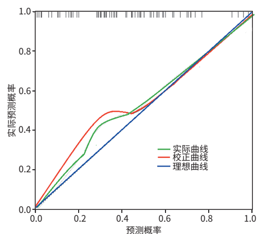
图7 验证组的校准曲线
