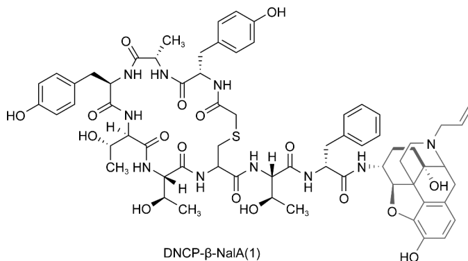
图9 DNCP- \beta -NalA (1)偶联物的化学结构式
