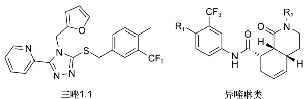
图 5 三唑类和异喹啉类 KOR 激动剂的化学结构式
