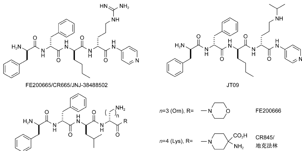
图6 外周选择性全D型-氨基酸四肽化学结构式
