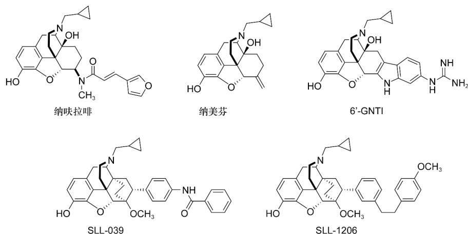
图 1 吗啡喃类 KOR 激动剂的化学结构式
