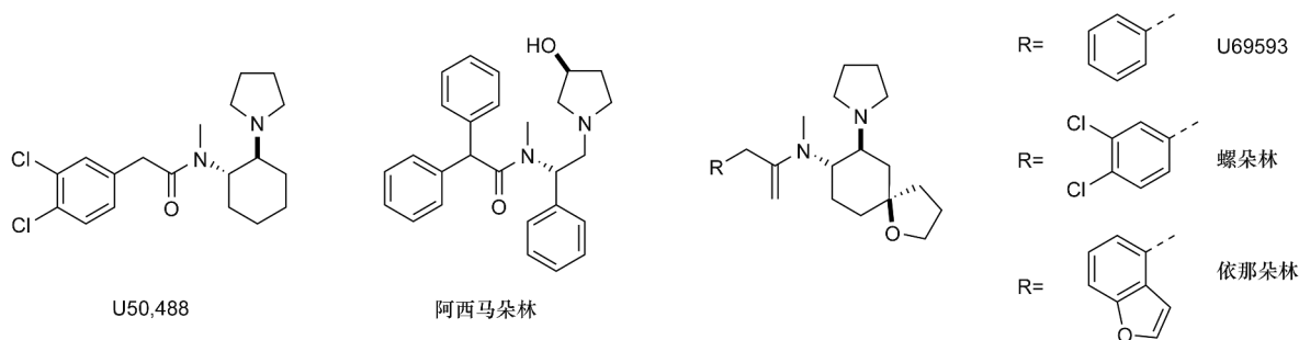
图 3 芳基乙酰胺类 KOR 激动剂的化学结构式
