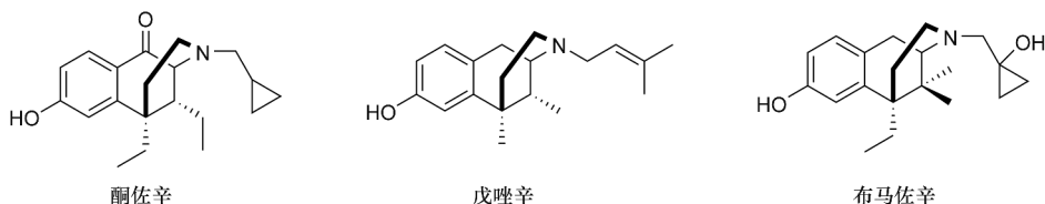
图 2 苯并吗啡烷类 KOR 激动剂的化学结构式
