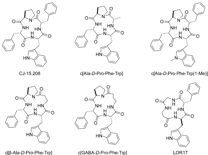
图8 大环四肽 CJ-15,208 及其衍生物的化学结构式
