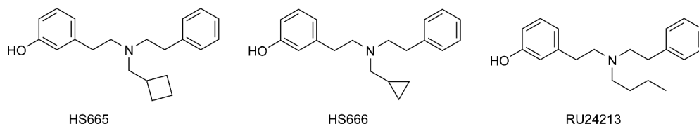
图 4 苯乙基胺类 KOR 激动剂的化学结构式
