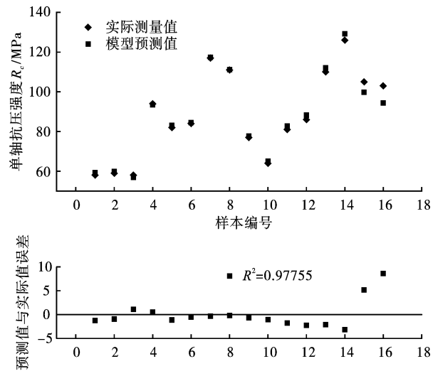
图 6 预测值与实际值误差 Fig. 6 Error of predicted and actual values
