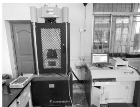
图 2 电脑控制电液伺服万能试验机
