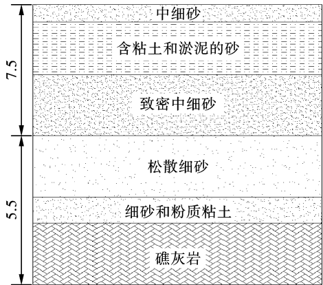
图 3 南卡罗来纳州爆炸压密试验场地 [24] (单位:m)
