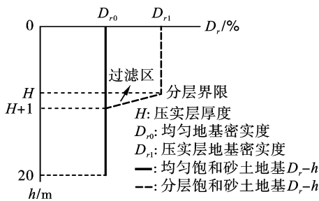
图 13 密实度随深度变化的简化计算图
