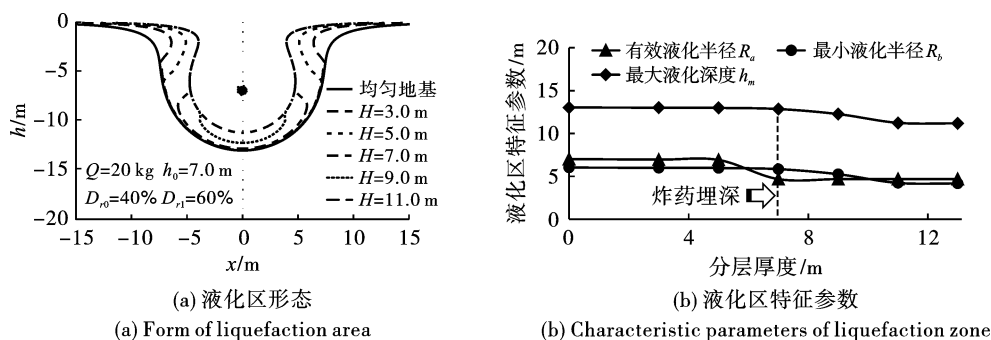
图 16 碾压密实层厚度对爆炸液化范围的影响
