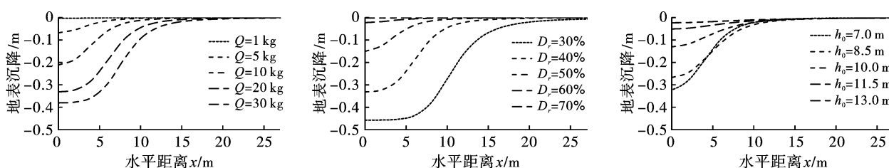
图10 均匀饱和砂土地基爆炸液化引起的地表沉降影响因素
