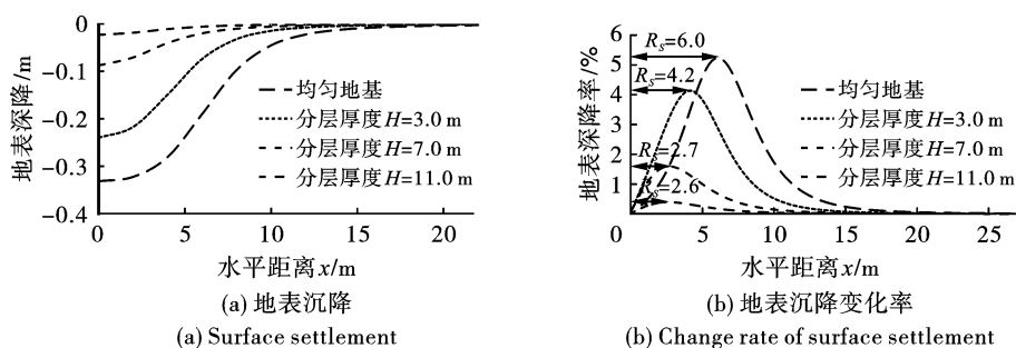
图 17 碾压密实层厚度对爆炸液化引起的地表沉降范围的影响
