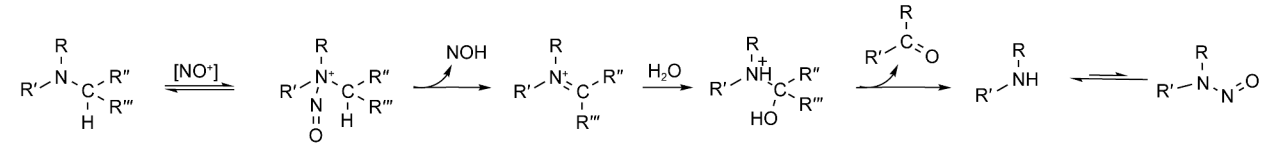
图 2 存在 α-H 的叔胺的亚硝化反应机制
