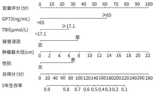
图 4 列线图模型
