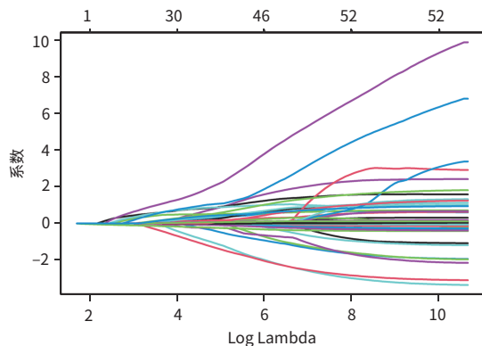
图1 Lasso回归参数选择
