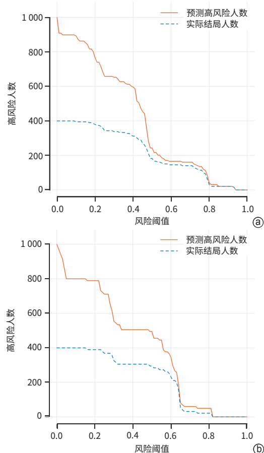
图7 临床影响曲线
