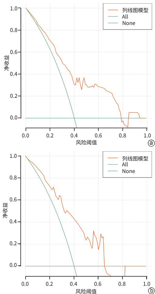
图6 临床决策曲线分析
