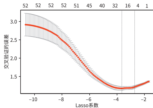
图2 交叉验证曲线
