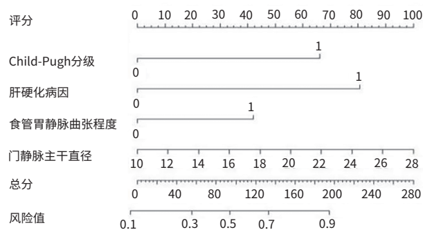
图3 预测模型的列线图
