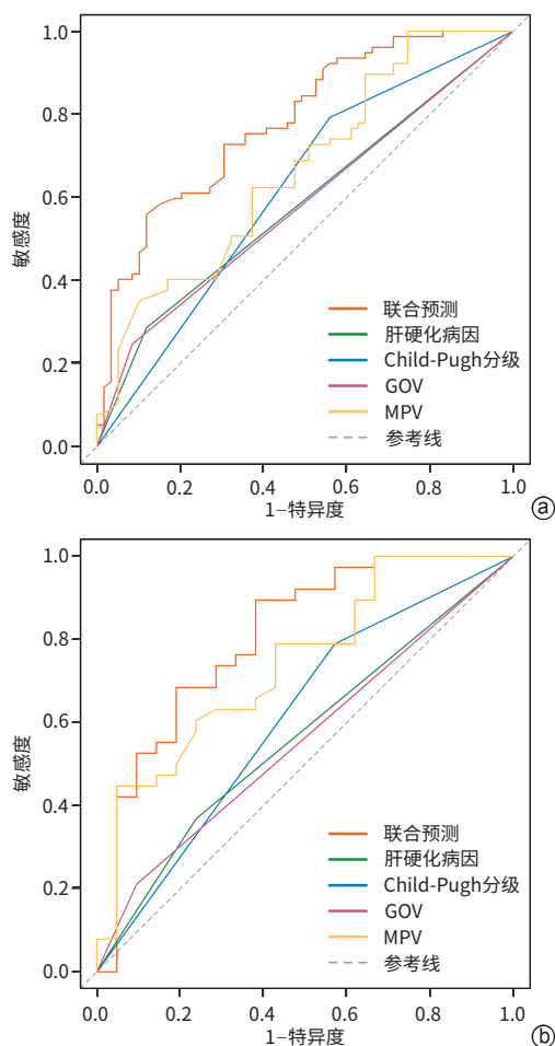
图4 受试者操作特征曲线
