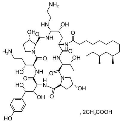
图1 醋酸卡泊芬净的化学结构式
