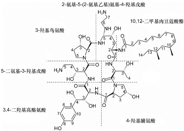
图 4 卡泊芬净的碳氢归属
