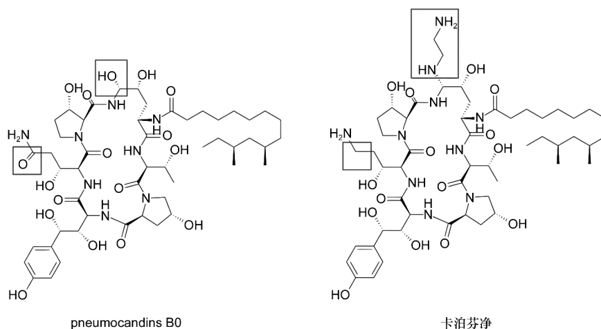
图3 pneumocandin B0 和卡泊芬净结构对比
