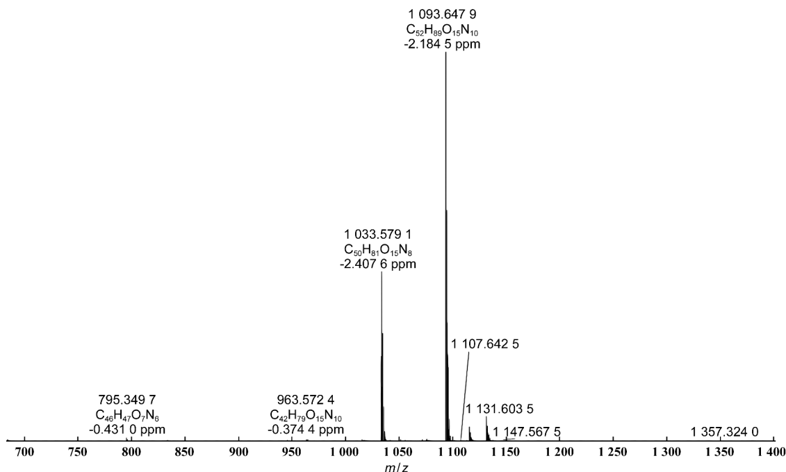
图2 醋酸卡泊芬净供试品质谱图
