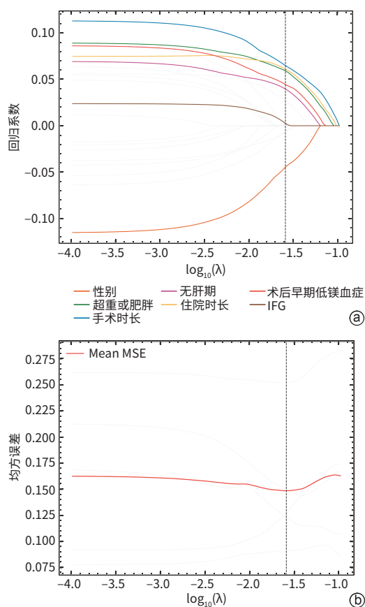
图1 Lasso回归分析
