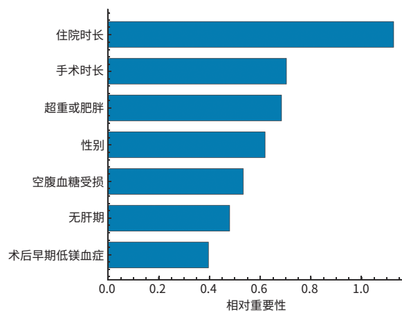
图5 XGBoost模型的特征重要性分析
